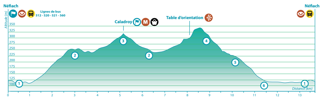
Profil topographique
