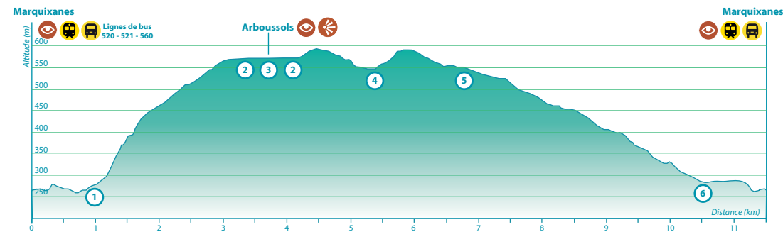
Profil topographique
